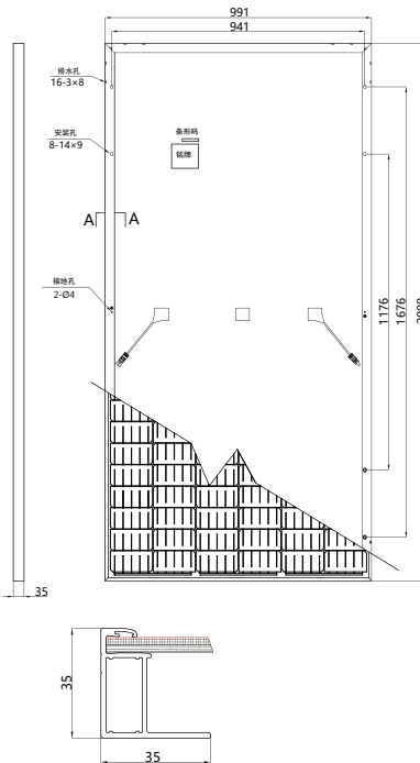
截面 A-A 尺寸 (单位: mm)
