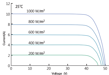
不同辐照度下电流电压曲线图
