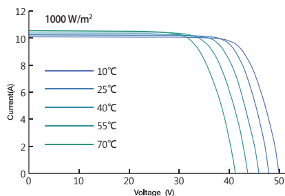
不同工作温度下电流电压曲线图
