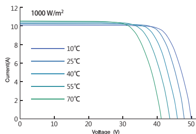
不同工作温度下电流电压曲线图
