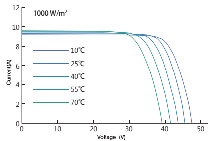
不同工作温度下电流电压曲线图
