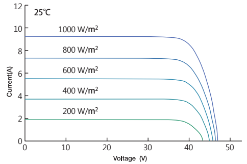
不同辐照度下电流电压曲线图
